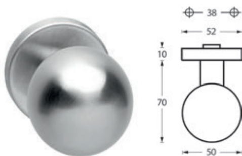
543-13 / vast Hartafstand: 38 mm Ø rozet: 52 mm Ø knop: 50 mm alleen bij vleugeloverdekkend paneel mogelijk! optioneel draaibaar
