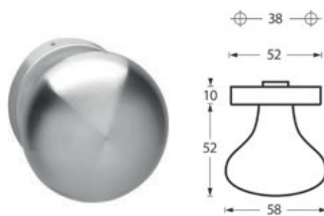
502-13 / vast Hartafstand: 38 mm Ø rozet: 52 mm Ø 58 mm alleen bij vleugeloverdekkend paneel mogelijk!
