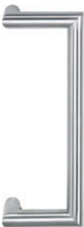
9043-13 Lengte: 380 mm Ø: 30 mm Hartafstand: 350 mm
